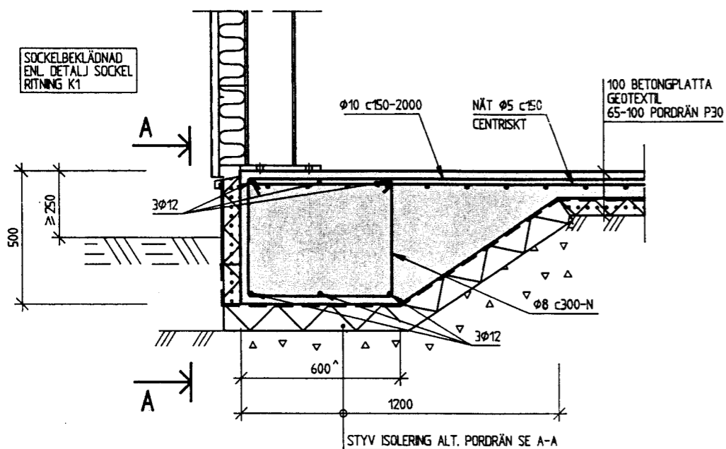
DETALJ 1: KANTBALK 1:20
