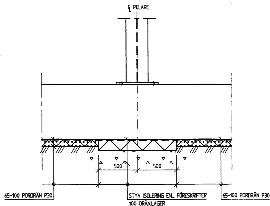
A-A 1:20
