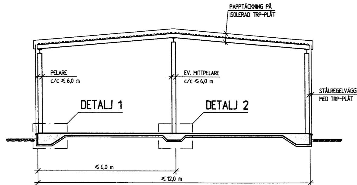
SEKTION A: INDUSTRIBYGGNAD 1 PLAN 1:100
